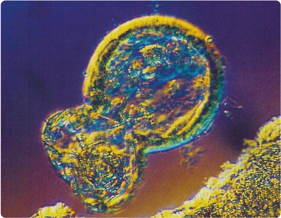
Embryon de gastéropode
